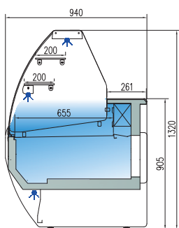
CVP-9-10-C CVP-9-13-C CVP-9-15-C CVP-9-20-C CVP-9-25-C CVP-9-30-C
