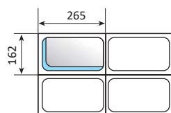
GN 1/4 162 X 265
