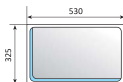
GN 1/1 325 X 530
