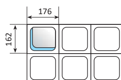
GN 1/6 176 X 162
